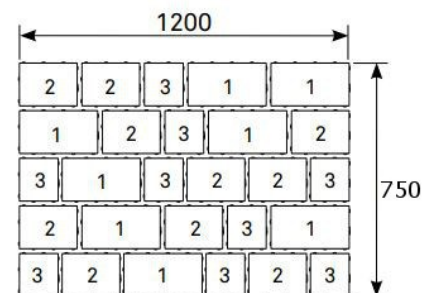
orientační skladba vrstvy
